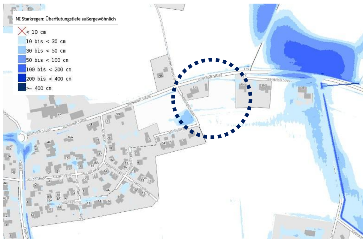
Außergewöhnliches Niederschlagsereignis (100-jährlich) © BKG
